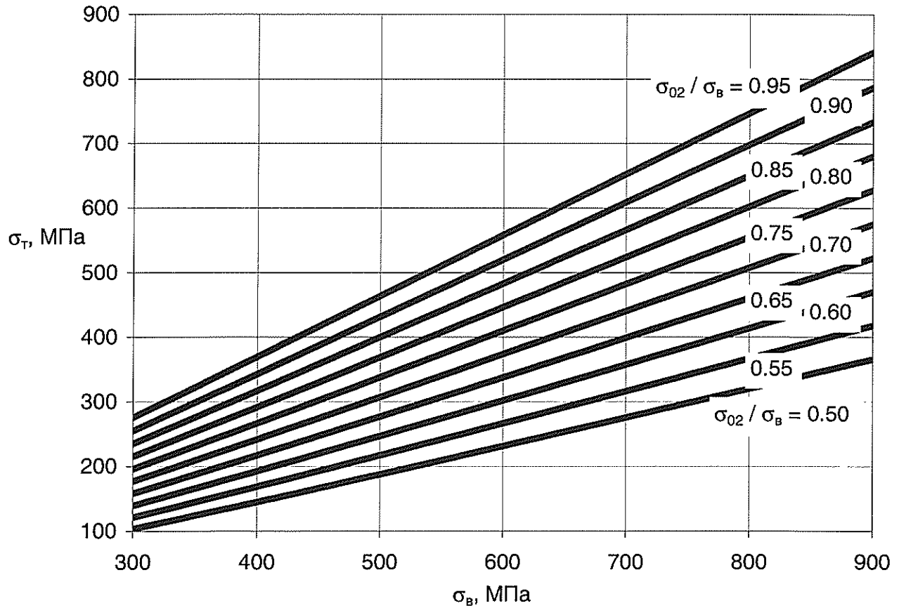
Рисунок 6 – Определение предела текучести \sigma_T
