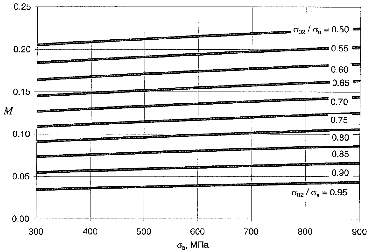
Рисунок 5 – Определение коэффициента деформационного упрочнения M
