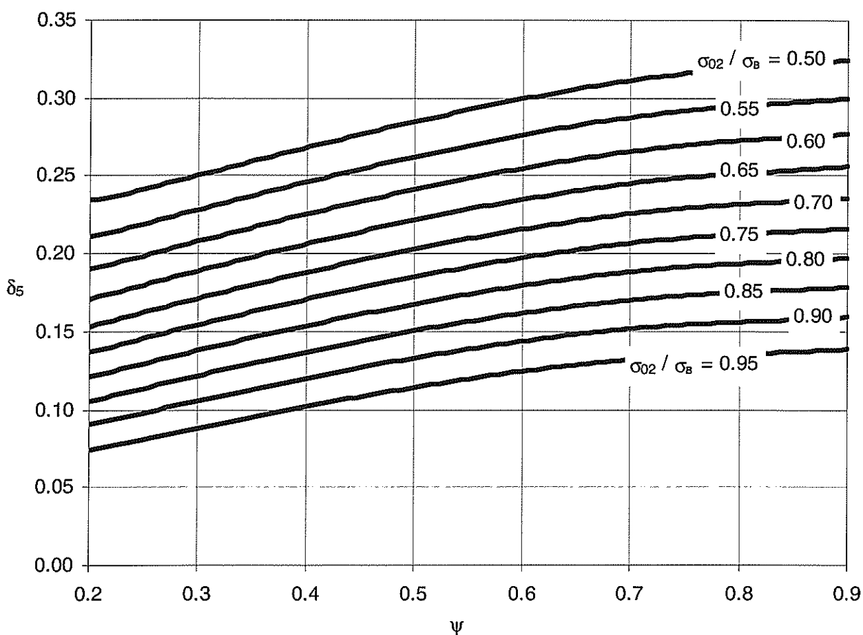
Рисунок 4 – определение относительного сужения после разрыва \psi
