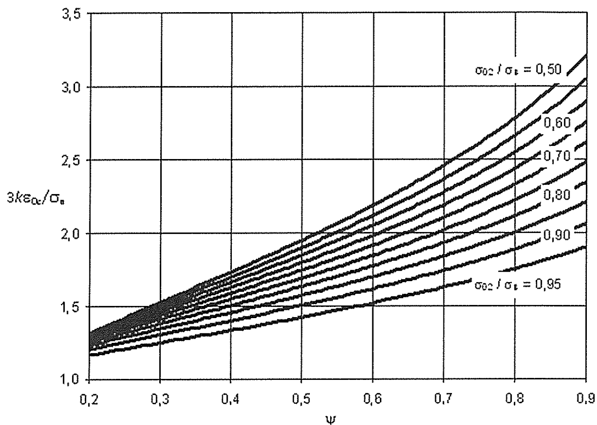
Рисунок 7 – Определение разрушающей объемной деформации \varepsilon_{0c}
