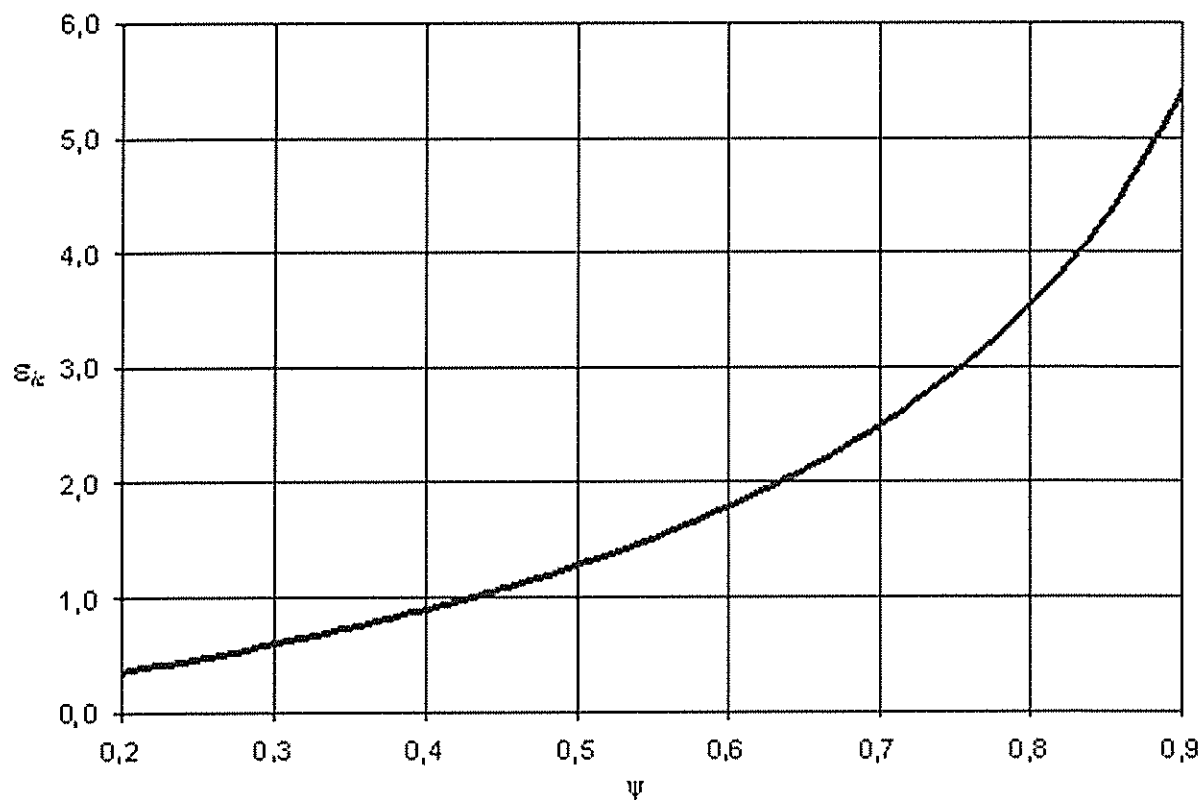
Рисунок 8 – Определение разрушающей интенсивности деформации \varepsilon_{0c}
