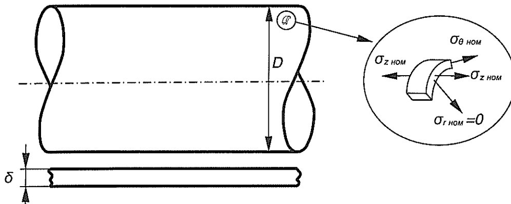
Рисунок 3 – Схема нагружения секции трубы
